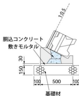
35-0.5 (控え350mm、勾配1:0.5用)
