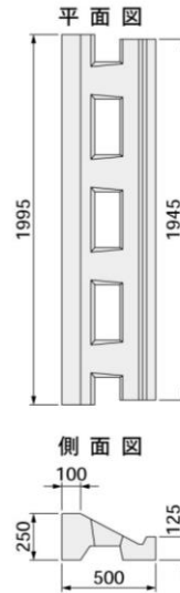
35-0.5 (控え350mm、勾配1:0.5用)
