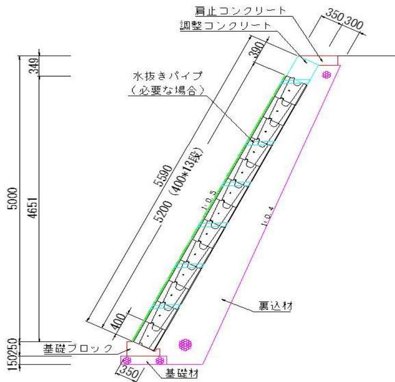
【標準断面図】
